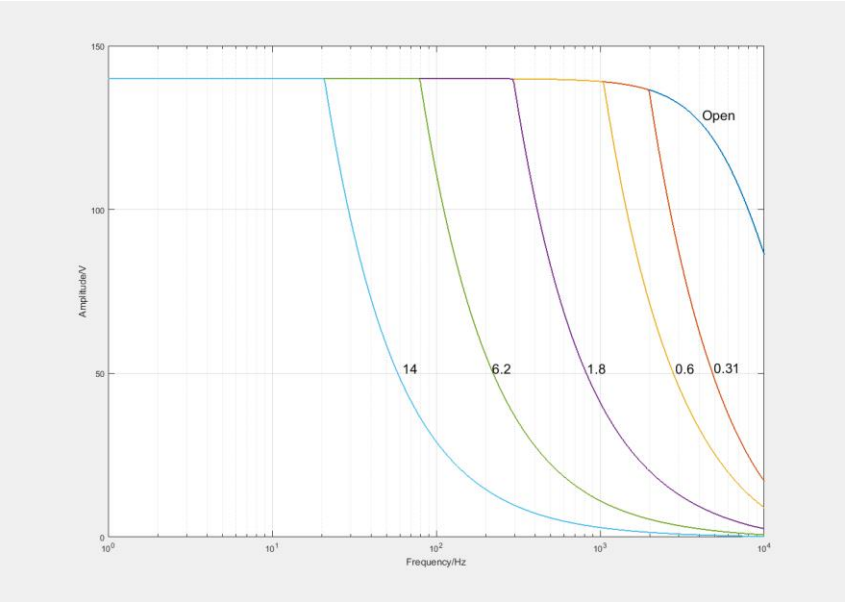
E-754 : 各种电容性负载的操作限制（开环），电容值的单位为微法
