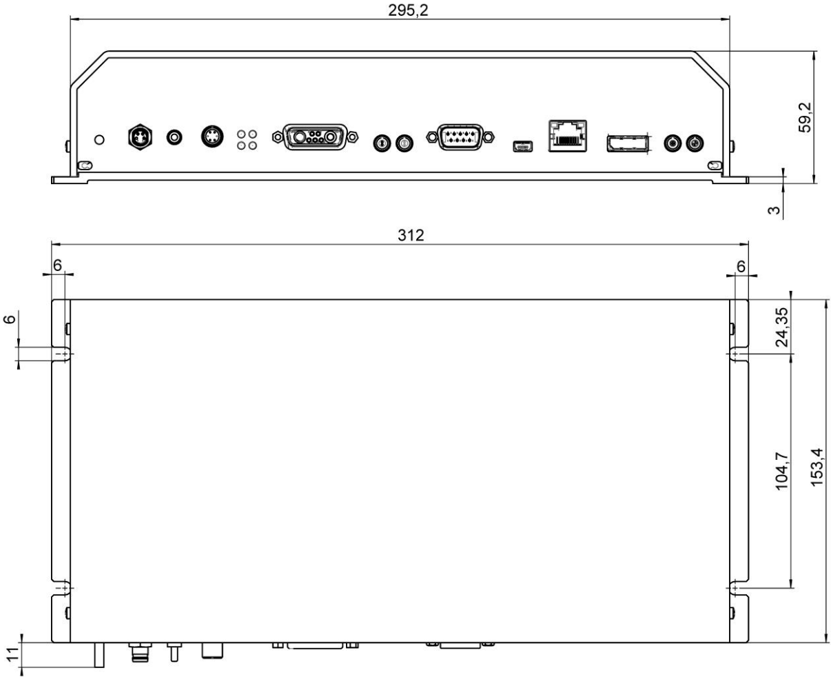
E-754, 尺寸单位是毫米
